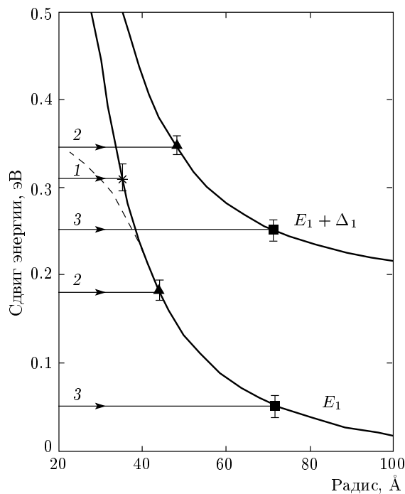
Рис. 5. Зависимости сдвигов энергии E_1, E_1 + \Delta_1 -резонанса от радиуса r цилиндра в плоскости роста. Сплошными линиями показаны зависимости, рассчитанные с помощью выражения (1). Символами обозначены положения резонансов, наблюдаемых в образцах с квантовыми точками германия. Горизонтальными стрелками 1, 2, 3 показаны проекции экспериментальных значений энергии резонанса на теоретические кривые. Эти значения получены из экспериментальных зависимостей, представленных на рис. 3, и обозначены теми же цифрами
