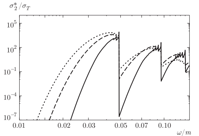
Рис. 3. То же, что и на рис. 2, для канала \gamma^{(2)}e \rightarrow e
