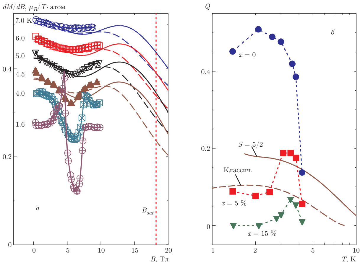
Рис. 6. (В цвете онлайн) а ) Сравнение экспериментально измеренной дифференциальной восприимчивости треугольного антиферромагнетика RbFe(MO_4)_2 (линии с символами из работы [10]) с вычислениями для модельного трехспинового кластера (сплошные кривые для квантовой модели, штриховые кривые — для классической модели). Температура Нееля для RbFe(MO_4)_2 в отсутствие внешнего поля приблизительно равна 4.3 К. Кривые для различных температур сдвинуты для наглядности, параметры модельной задачи подобраны по низкотемпературным полю насыщения и намагниченности, как описано в тексте. б ) Сравнение определенного из эксперимента фактора качества плато для Rb_{1-x}K_xFe(MO_4)_2 (кривые с символами из работы [14]) с вычислениями для модельного трехспинового кластера (сплошные кривые для квантовой модели, штриховые кривые для классической модели). Параметры модельной задачи подобраны, как описано в тексте
