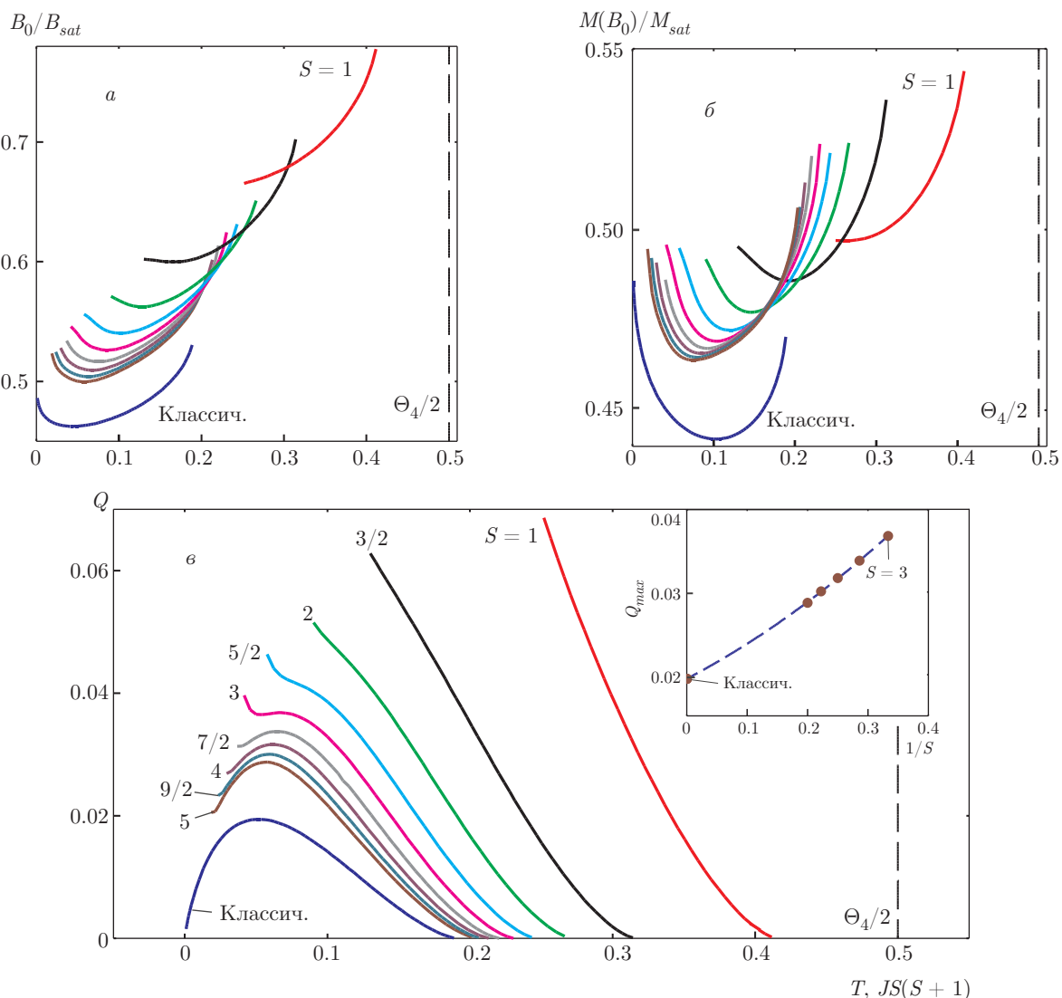
Рис. 5. (В цвете онлайн) Параметры напоминающей плато особенности на кривых намагничивания для четырехспинового ( N = 4 ) кластера спинов S \geq 1 (включая классический предел): a — температурная зависимость положения минимума дифференциальной восприимчивости; б — температурная зависимость величины полной намагниченности кластера в поле минимума дифференциальной восприимчивости; в — температурная зависимость фактора качества плато, на вставке: зависимость максимального значения фактора качества плато от спина в вершине кластера для S \geq 3 , штриховая проведена для наглядности. Все панели используют одинаковую цветовую схему для маркировки кривых. Вертикальные штриховые линии на рис. a, б, в отмечают значения половины температуры Кюри–Вейса, для квантовой модели шкала температур выражена в единицах JS(S + 1) , для классических моделей — в единицах J
