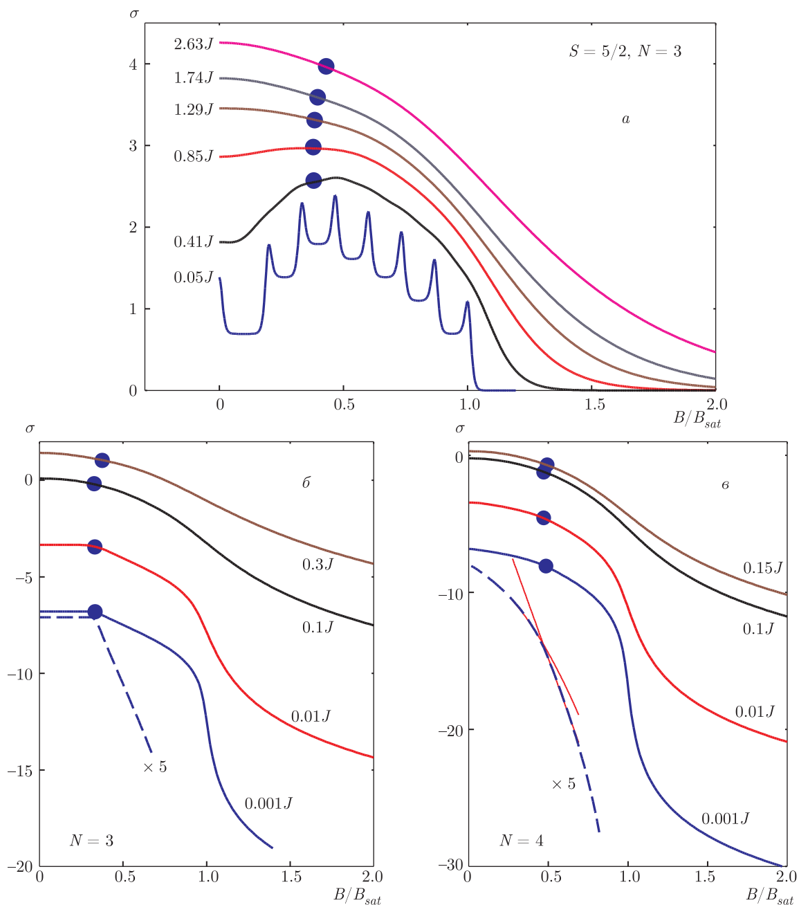
Рис. 3. (В цвете онлайн) Полевые зависимости энтропии при различных температурах для трехспиновой кластера квантовых спинов S = 5/2 (a) и трех- и четырехспиновой кластера классических спинов (б, в). Темные кружки отмечают положения минимума дифференциальной восприимчивости при соответствующей температуре. Штриховые кривые (для классических моделей на рис. б, в) показывают соответствующие кривые после растяжения в 5 раз вдоль оси Y для более наглядной демонстрации изменения наклона кривых \sigma(B) , тонкие красные линии на рис. в являются гладкими кривыми, проведенными через точки кривой \sigma(B) выше и ниже изменения наклона, их пересечение отмечает точку изменения наклона. Значения температуры на рис. а в единицах JS(S+1) равны, соответственно, 0.0057, 0.0463, 0.097, 0.148, 0.199 и 0.3
