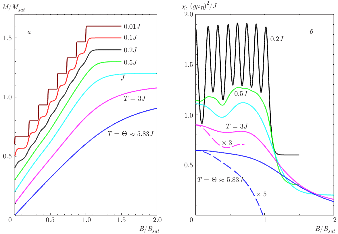
Рис. 1. (В цвете онлайн) a ) Кривые намагничивания для трехспинового кластера спинов S = 5/2 при различных температурах, кривые смещены для наглядности; б ) полевые зависимости дифференциальной восприимчивости для трехспинового кластера спинов S = 5/2 при различных температурах, кривые смещены для наглядности. Штриховые кривые на рис. б увеличены по оси Y с указанным коэффициентом
