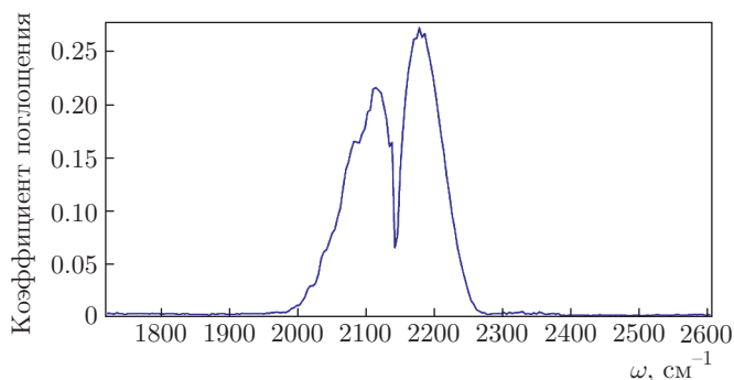
Рис. 1. Колебательно-вращательный спектр молекулы CO [5]
