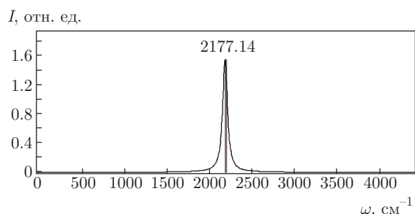
Рис. 2. Колебательно-вращательный спектр поглощения молекулы CO, полученный с помощью матрицы Гессе
