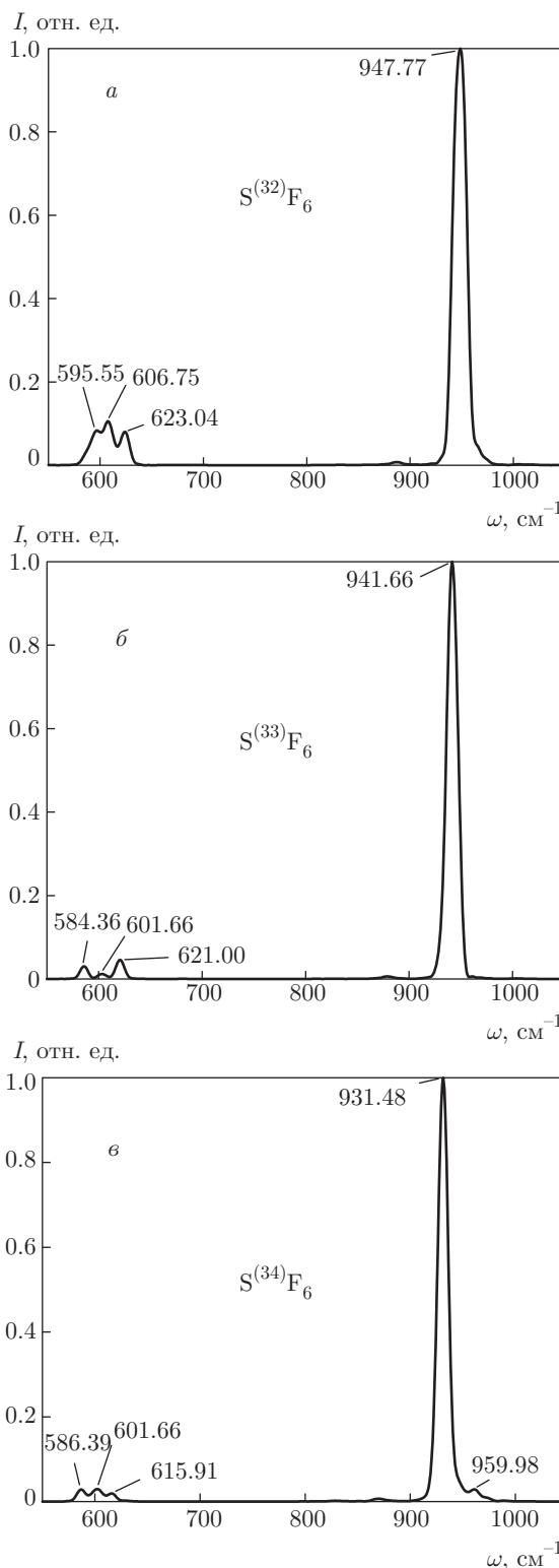
Рис. 4. Колебательно-вращательные спектры поглощения мономеров S (32) F 6 (а), S (33) F 6 (б) и S (34) F 6 (в)
