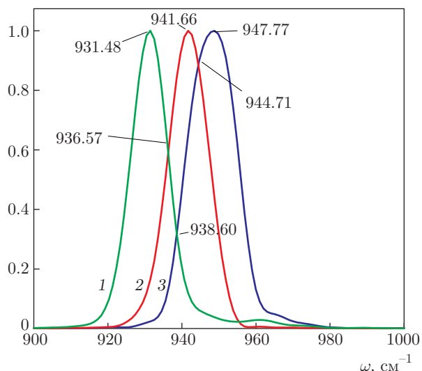
Рис. 5. Влияние массы атома S на канал \nu_3 колебательно-вращательного спектра поглощения мономера \text{SF}_6 : кривая 1 — S^{(32)} ; 2 — S^{(33)} ; 3 — S^{(34)} . Спектральное разрешение 1.02 \text{ см}^{-1}
