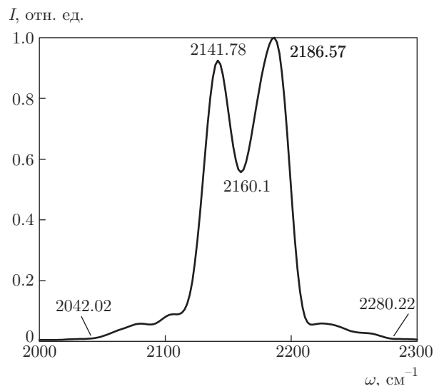
Рис. 3. Расчетный колебательно-вращательный спектр поглощения молекулы CO по данным метода молекулярной динамики
