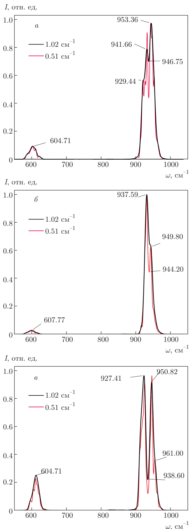
Рис. 6. (В цвете онлайн) Колебательно-вращательные спектры поглощения гомодимеров S^{(32)}F_6-S^{(32)}F_6 (а) и гетеродимеров S^{(32)}F_6-S^{(33)}F_6 (б), S^{(32)}F_6-S^{(34)}F_6 (в)
