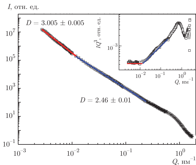
Рис. 1. (В цвете онлайн) Малоугловое рассеяние нейтронов на ядрах куриных эритроцитов. Интенсивность рассеяния нейтронов в диапазоне переданных импульсов 10^{-3} – 10^{-2} нм ^{-1} — данные установки TPA LLB, Сакле, Франция. Интенсивность рассеяния нейтронов в диапазоне переданных импульсов 10^{-2} – 10^0 нм ^{-1} — данные установки PA20 LLB, Сакле, Франция
