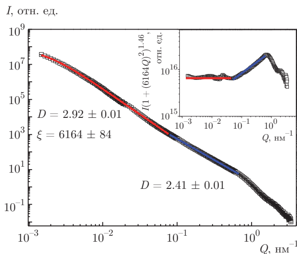
Рис. 2. (В цвете онлайн) Малоугловое рассеяние нейтронов на ядрах HeLa. Интенсивность рассеяния нейтронов в диапазоне переданных импульсов 1.5 \cdot 10^{-3} – 2 \cdot 10^{-2} нм ^{-1} — данные установки KWS-3, MLZ, Гархинг, Германия. Интенсивность рассеяния нейтронов в диапазоне переданных импульсов 2 \cdot 10^{-2} – 3 \cdot 10^0 нм ^{-1} — данные установки D11, ILL, Гренобль, Франция
