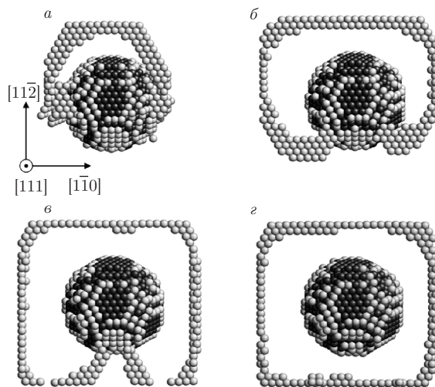
Рис. 2. Визуализация процесса роста дислокационной петли при сдвиговой деформации \epsilon_{yz} ( \gamma = 0.1 рад). Температура расчетной ячейки 300 К. Представлены результаты через 1.25 пс (а), 2.5 пс (б), 3.75 пс (в), 5 пс (г). Частицы, выделенные темным цветом, образуют поверхность поры
