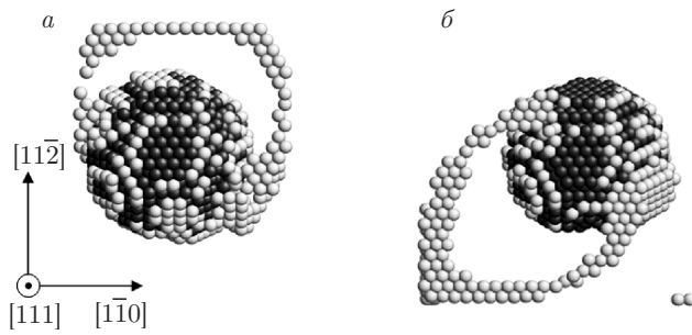
Рис. 4. Визуализация частичных дислокационных петель, образующихся под воздействием ударных волн, при сдвиговых деформациях \varepsilon_{xz} (а) и \varepsilon_{yz} (б) ( \gamma = 0.06 рад). Температура расчетной ячейки 300 К
