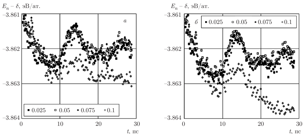
Рис. 1. Зависимости изменения потенциальной энергии моделируемой системы (представлены сопоставленные значения) от времени при различных углах \gamma [рад]. Температура расчетной ячейки 300 К. Представлены результаты для сдвиговых деформаций \epsilon_{xz} (а) и \epsilon_{yz} (б)
