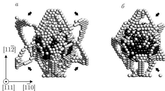
Рис. 5. Визуализация частичных дислокационных петель (а), образование которых осуществляется после прохождения ударной волны, и дислокаций Ломер–Коттрела (б), сформировавшихся в процессе релаксации структуры. Температура расчетной ячейки 600 К. Сдвиговая деформация \varepsilon_{yz} ( \gamma = 0.06 рад)
