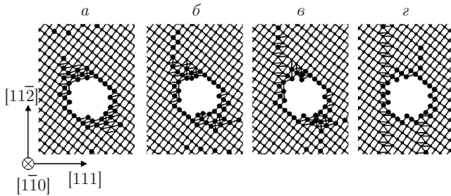
Рис. 3. Визуализация плоскости (\bar{1}\bar{1}0) расчетной ячейки при сдвиговой деформации \varepsilon_{yz} ( \gamma = 0.1 рад) через 1.25 пс (а), 1.75 пс (б), 2.5 пс (в), 7.5 пс (г). Для наглядности выделены частицы, энергия связи которых отлична от энергий большинства частиц ячейки
